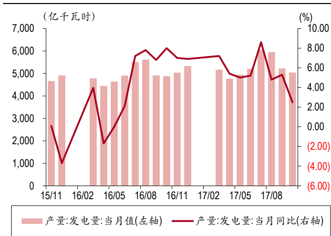
图表 114. 全国发电量同比+2.50%
