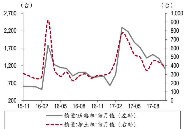
图表 48. 压路机和推土机销量继续走低
