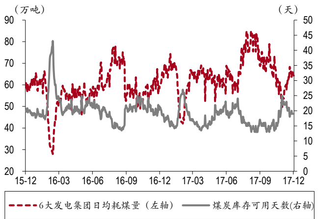
图表 13. 6 大发电集团日均耗煤量持续走高
